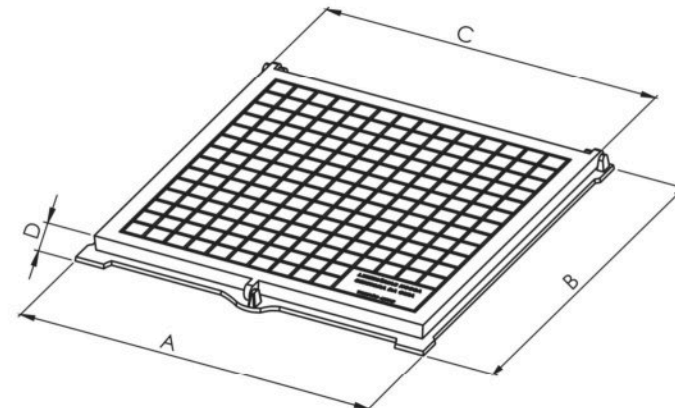
TAMPÃO SIMPLES 40X40 CM TAMPÃO REFORÇADO 40X40 CM
