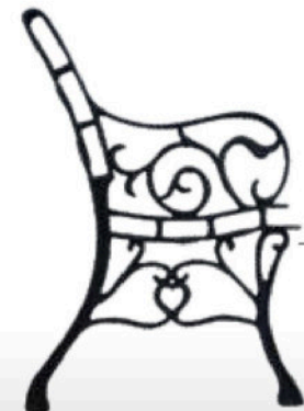
PE DE BANCO FRANCES BC 245 Alt.: 76 cm Alt. Assento: 38 cm Larg.: 54 cm
