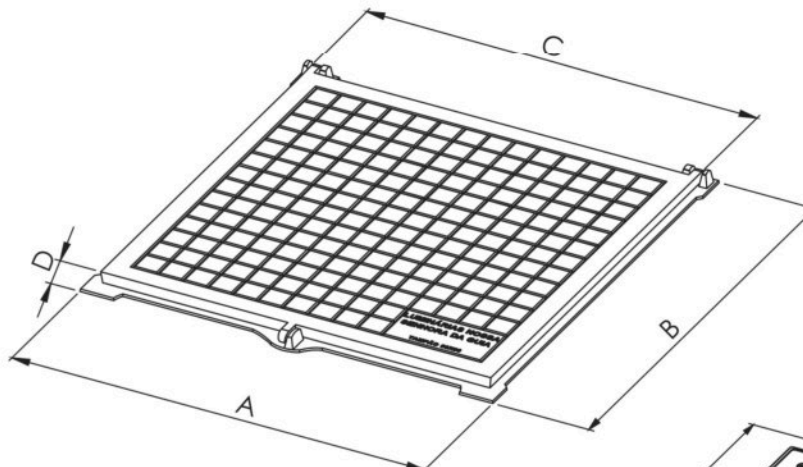
TAMPÃO SIMPLES 60X60 CM TAMPÃO REFORÇADO 60X60 CM
