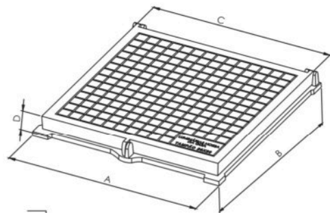
TAMPÃO SIMPLES 20X20 CM
